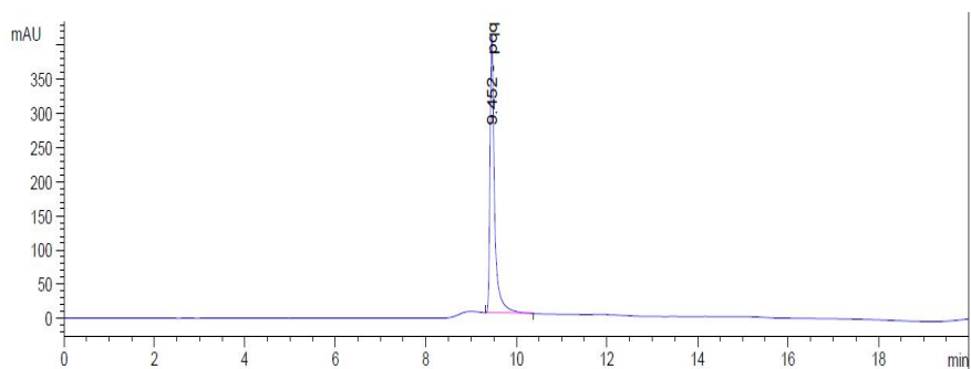
图 A.2 吡咯并喹啉酮二钠标准品液相色谱图
