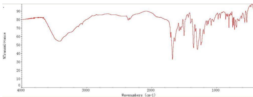
图 A.1 吡咯并喹啉酮二钠标准品红外光谱图
